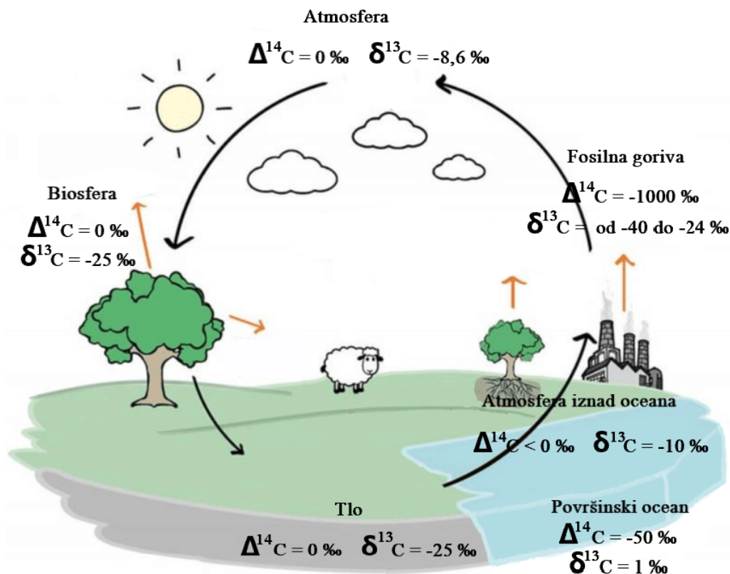
Slika 3.4: Ciklus ugljika s \Delta^{14}\text{C} i \delta^{13}\text{C} vrijednostima različitih spremnika ugljika.
