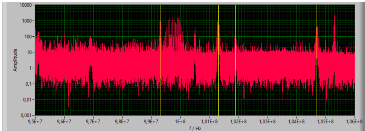
Slika 7.3. Amplitudni spektar signala između frekvencija 95 MHz i 106 MHz
