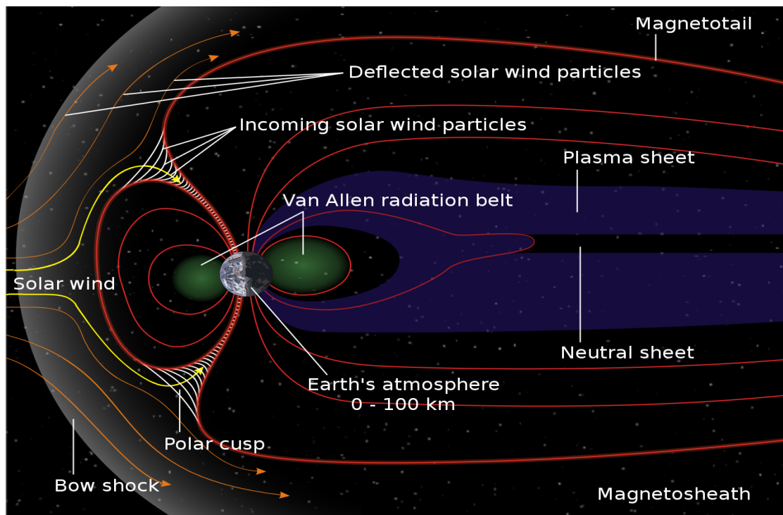
Slika 2.6: Zemljina magnetosfera [6]
