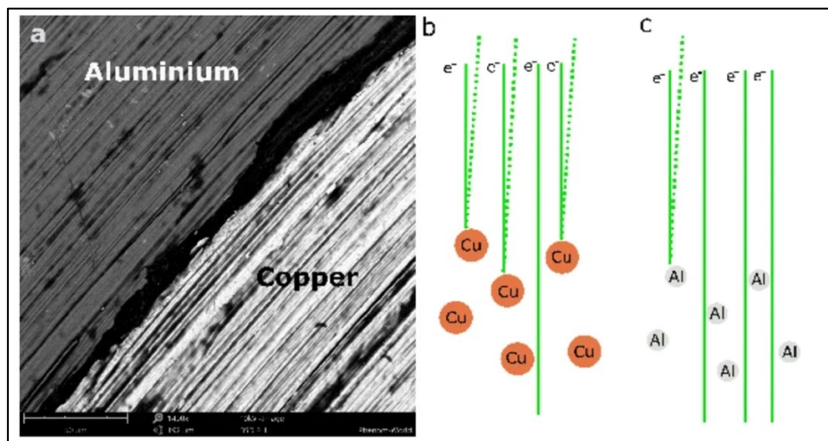
Slika 2.9. a) SEM slika uzorka koji sadrži aluminij i bakar nastala pomoću povratno raspršenih elektrona, ilustracija međudjelovanja primarnih elektrona s atomima b) bakra i c) aluminijski i nastanak povratno raspršenih elektrona [10]
