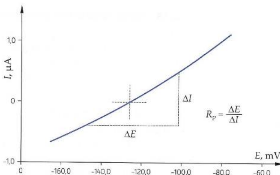
Slika 7.3 Princip određivanja polarizacijskog otpora ili otpora Faradayevoj reakciji [21]
