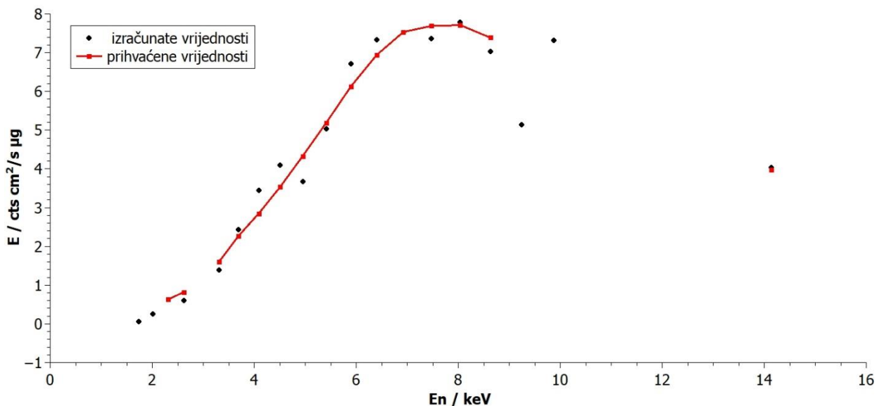
Slika 3.3 Elementne efikasnosti XRF sustava i prilagodba glatkom krivuljom.
