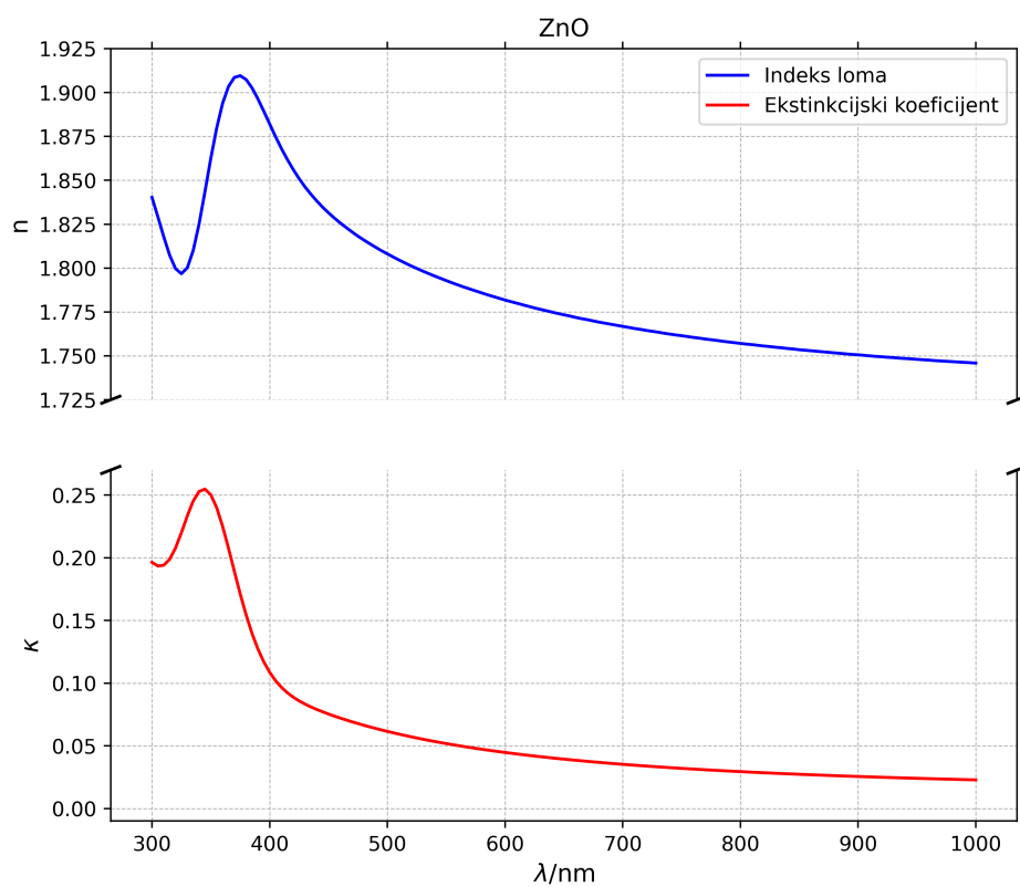
Slika 6: Indeks loma i ekstinkcijski koeficijent za ZnO u ovisnosti o valnoj duljini. Podaci preuzeti iz [5].
