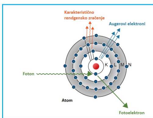
Slika 3.1. Fotoelektrični učinak [6]
