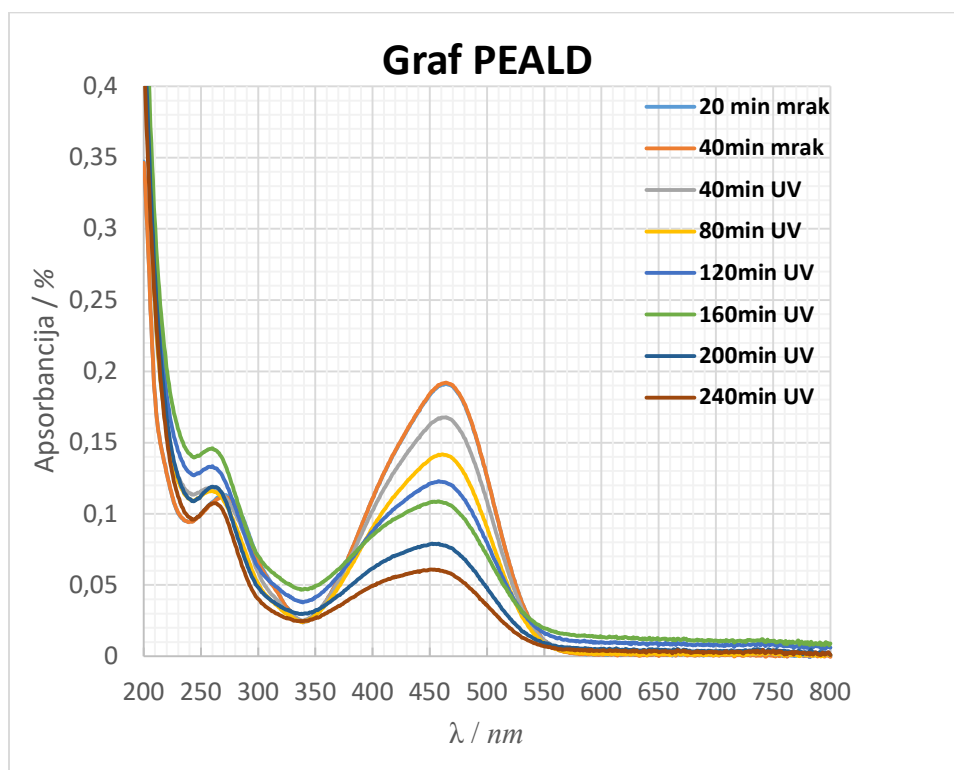
Slika 4.1.2 PEALD
