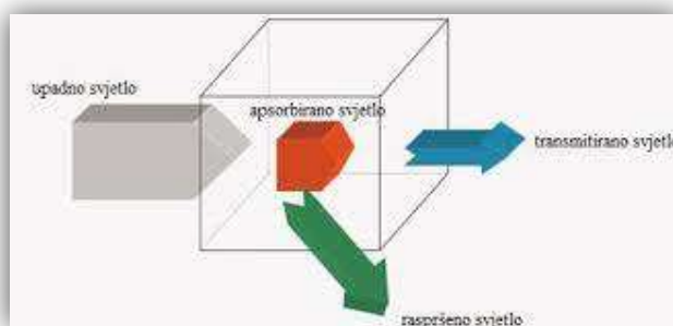
Slika 2.1.2. Prolazak svjetlosti [6]
