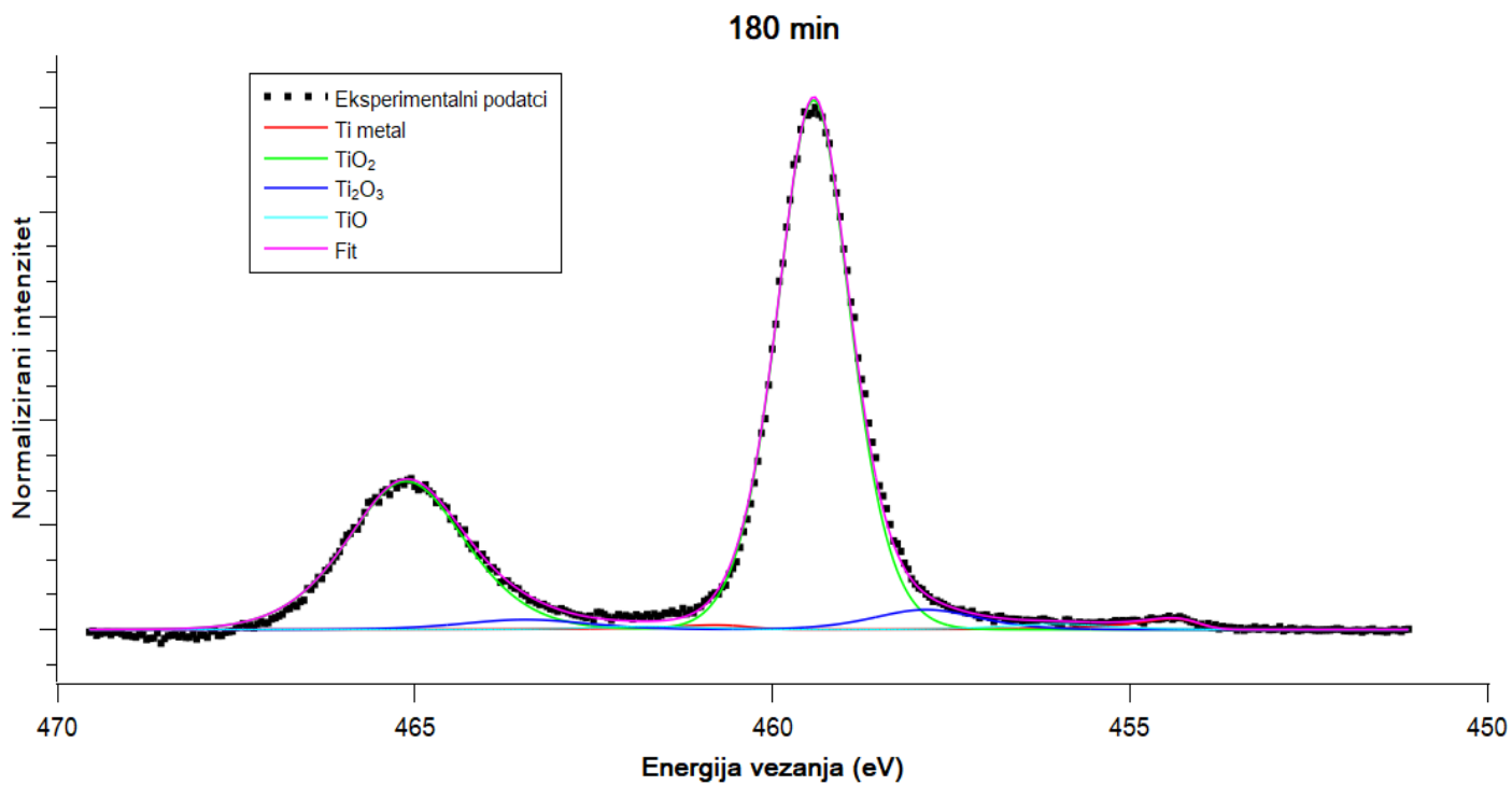
Slika 6.2. Fotoemisijski spektri oko Ti 2p atomskih nivoa uzorka titana bombardiranih s ionima O_2^+ energije 1 keV za različita vremena bombardiranja. Eksperimentalni spektri su prikazani s točkama, dok pune linije prikazuju numeričku prilagodbu pomoću produkta Gaussovih i Lorentzovih krivulja.
