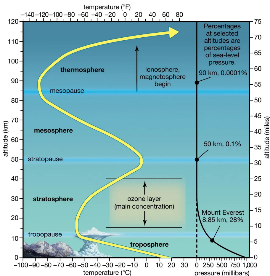
Slika 2.1: Vertikalni presjek Zemljine atmosfere [26].
