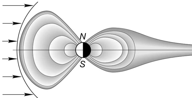
Slika 1.2: Shematski prikaz magnetskog polja planeta [8]. Strelice slijeva – Sunčev vjetar, N (engl. north ) – sjeverni pol, S (engl. south ) – južni pol.
