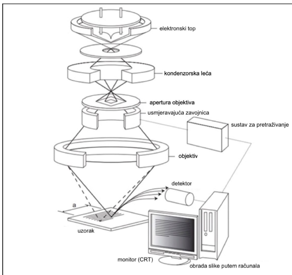
Slika 2.1. Shematski prikaz SEM-a [3]
