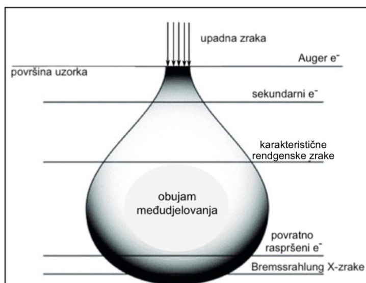
Slika 2.6. Obujam međudjelovanja [9]
