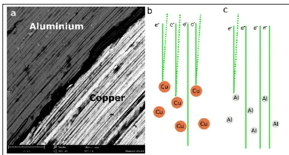
Slika 2.9. a) SEM slika uzorka koji sadrži aluminij i bakar nastala pomoću povratno raspršenih elektrona, ilustracija međudjelovanja primarnih elektrona s atomima b) bakra i c) aluminijskog i nastanak povratno raspršenih elektrona [10]
